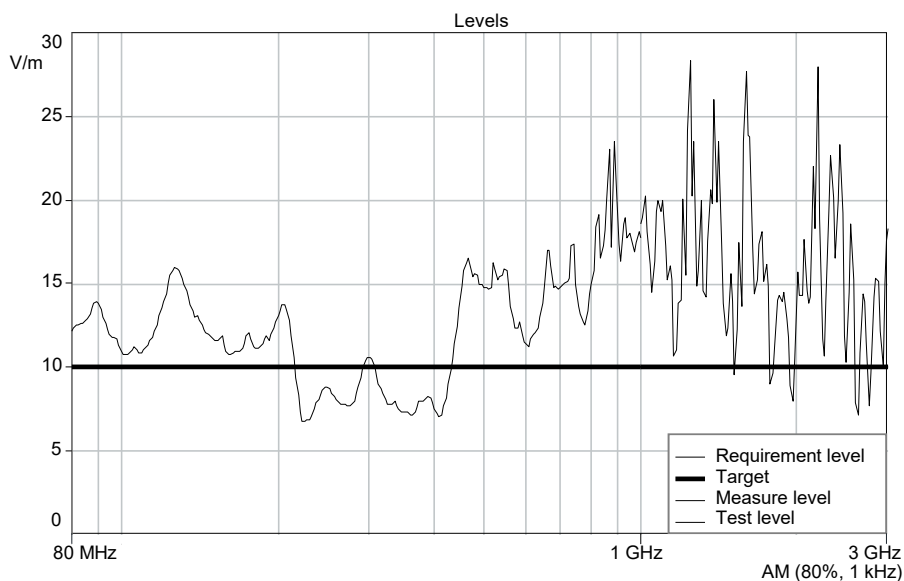
Abbildung 15: Prüfpegel und Monitoring während dem Test der Störfestigkeit gegen elektromagnetische Felder
