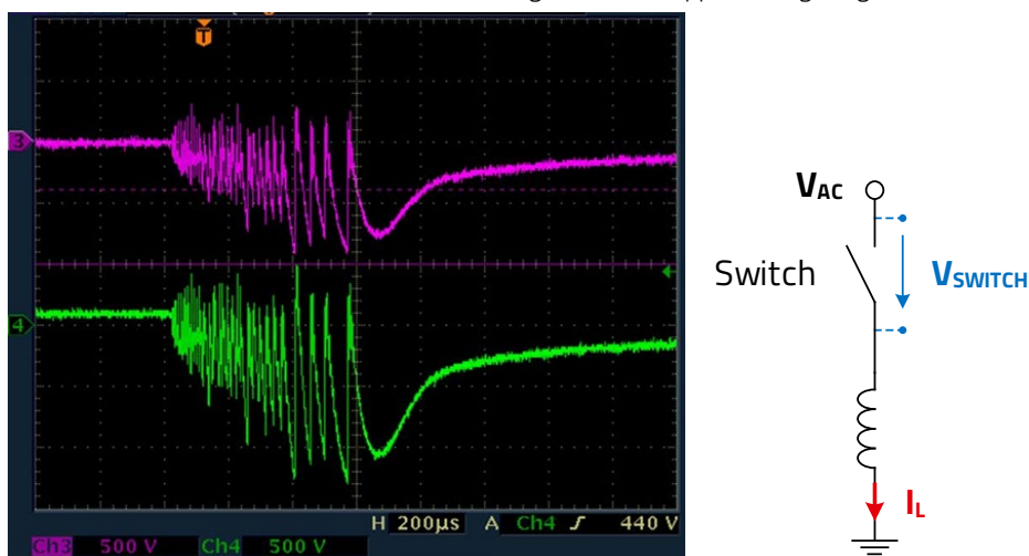
Abbildung 17: Entstehung eines Burstpakets in einer realen Applikation
