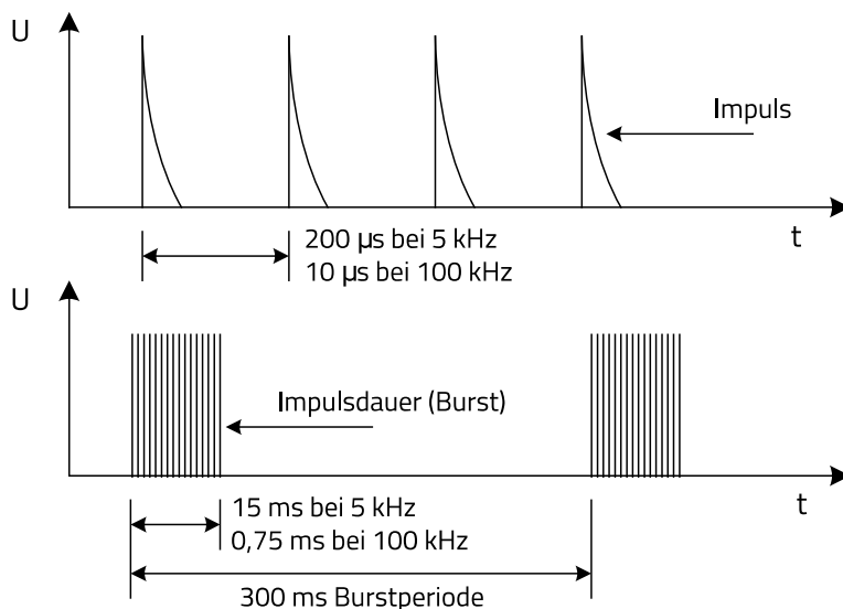
Abbildung 18: Prüfsignal zur Prüfung der Immunität gegen Burst nach DIN EN 61000-4-4:201404
