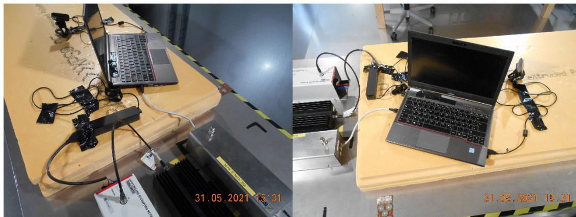
Abbildung 26: Aufbau der leitungsgeföhrt Störfestigkeitsprüfung am Notebook
