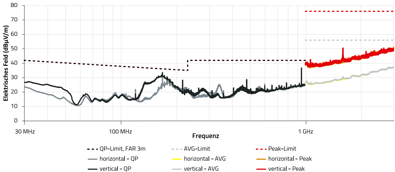
Abbildung 9: Gestrahlte Störaussendungsprüfung des Prüfaufbaus aus Abbildung 8
