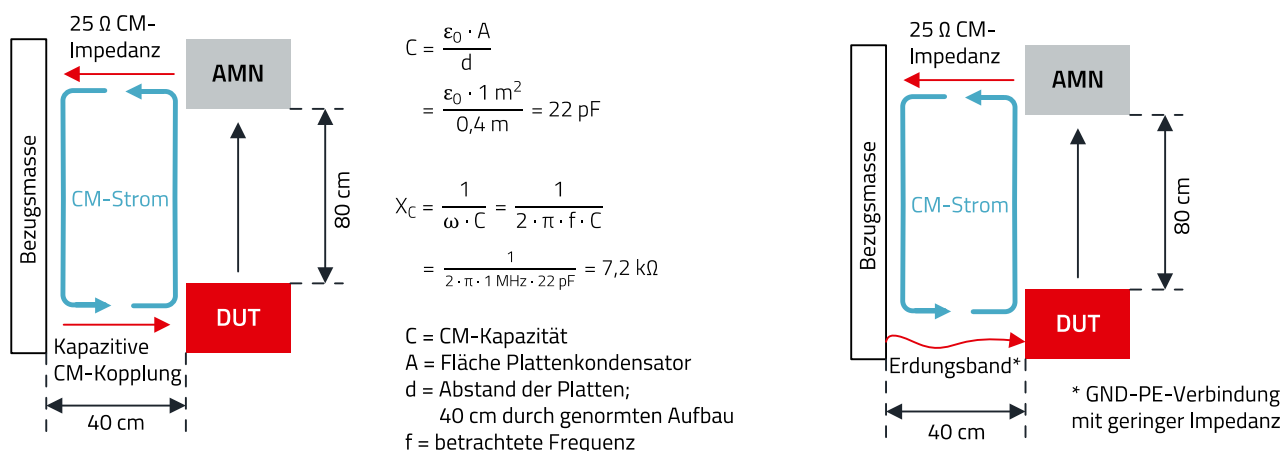
Abbildung 4: Verhalten Common Mode Loop, wenn ein Kabelschirm im Prüfaufbau hart geerdet wird
