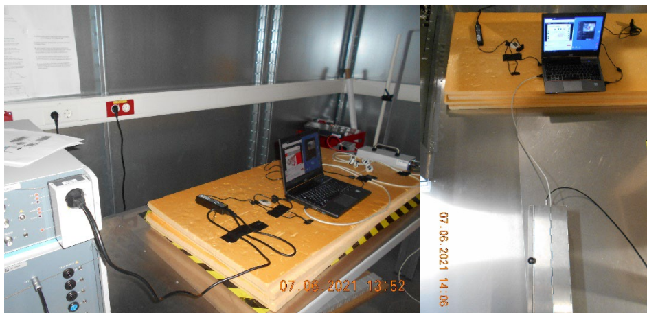
Abbildung 20: Aufbau der Prüfung der Störfestigkeit gegen schnelle Transiente (Burst). Links der Aufbau der Prüfung an der Schnittstelle zum Niederspannungsnetz, rechts an der Datenleitung
