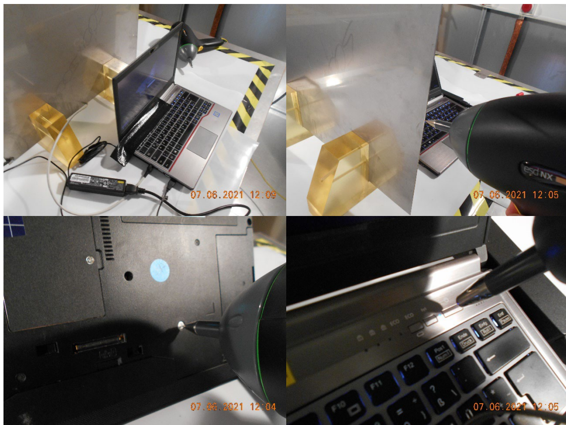
Abbildung 11: Prüfaufbau zur ESD-Prüfung des Notebooks. Prüfung an einer metallischen Schraube mit direkter ESD-Entladung (unten links) und indirekter Entladung am Haupttaster (unten rechts). ESD-Entladung auf VCP (oben rechts) und Gesamtübersicht des Prüfaufbaus (oben links)
