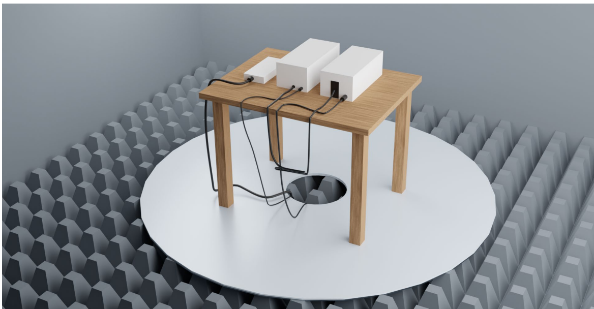
Abbildung 7: Bild D.11 der DIN EN 55032:2016 zeigt den schematischen Aufbau der gestrahlten Störaussendungsprüfung in einem Vollabsorberraum
