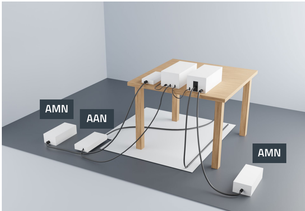
Abbildung 2: Bild D.2 in CISPR 32:2016 zeigt den schematischen Aufbau der leitungsgeführten Störaussendungsprüfung
