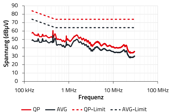
Abbildung 6: Messung der Störspannung nach der AAN-Methode auf dem Kabelschirm des Ethernetkabels
