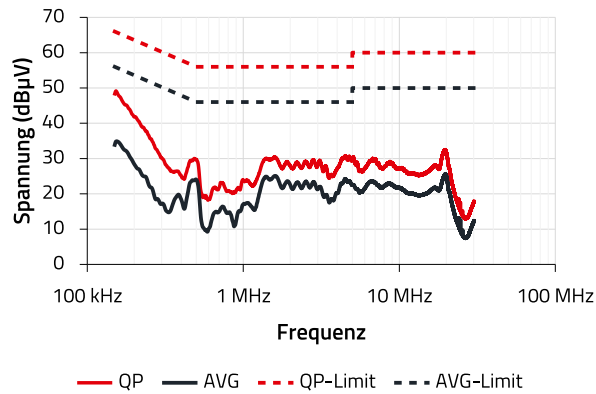
Abbildung 5: Messergebnis der leitungsgeführten Störaussendungsprüfung am Anschluss zum Niederspannungsnetz
