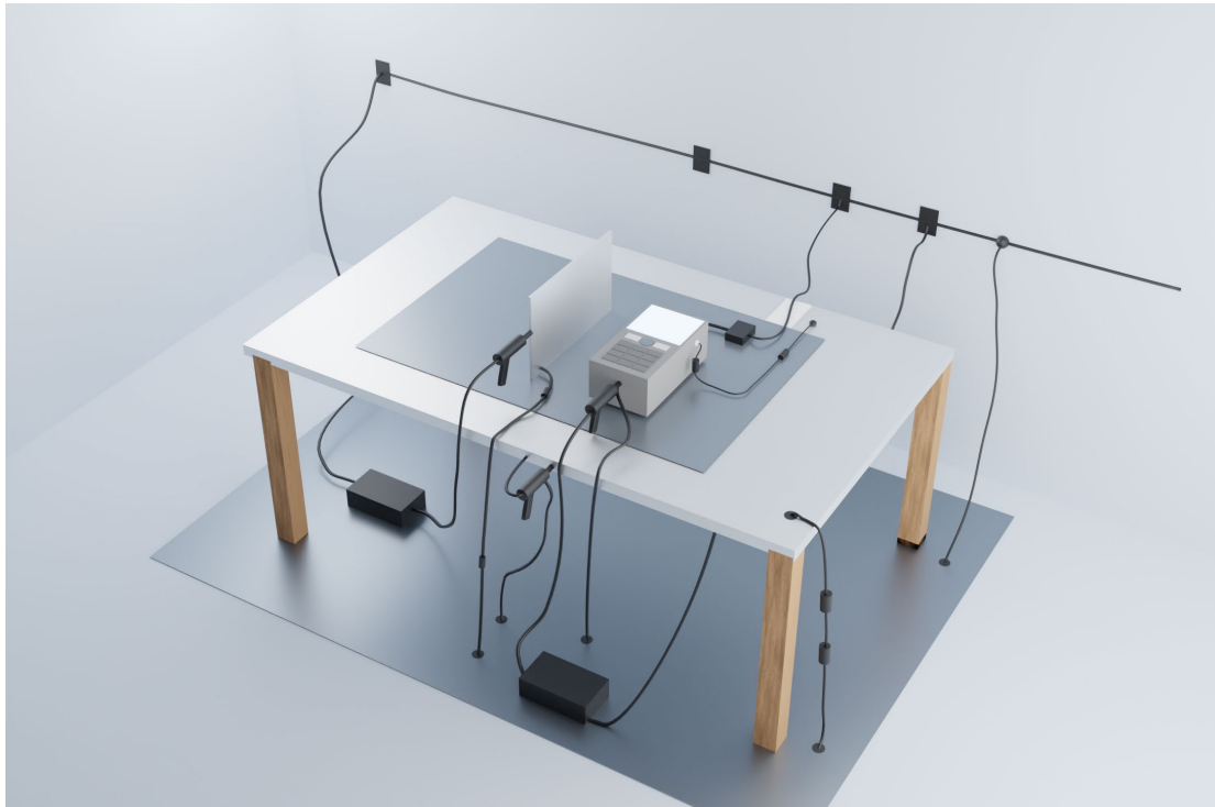
Abbildung 10: normativer, schematischer Prüfaufbau der ESD-Störfestigkeitsprüfung nach DIN EN 61000-4-2_2009-12
