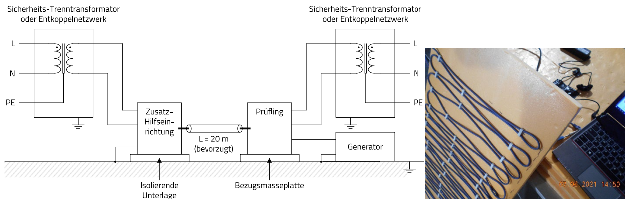
Abbildung 23: Surgeprüfung auf geschirmtem Ethernetkabel. Links der normative Aufbau nach DIN EN 61000-4-5:2014+A1:2017; Rechts Umsetzung des Aufbaus mit Einkopplung auf 20 m langem mäandriertem geschirmtem Kabel
