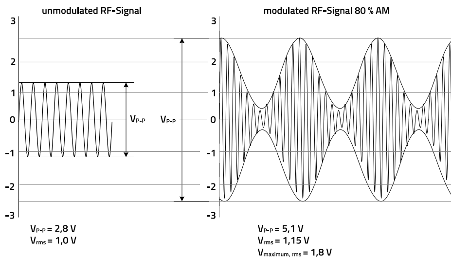
Abbildung 12: Prüfsignal zur Prüfung der leitungsgeführten und gestrahlten Störfestigkeit. Abbildung entstammt der IEC 61000-4-3:2006+A1:2007+A2:2010
