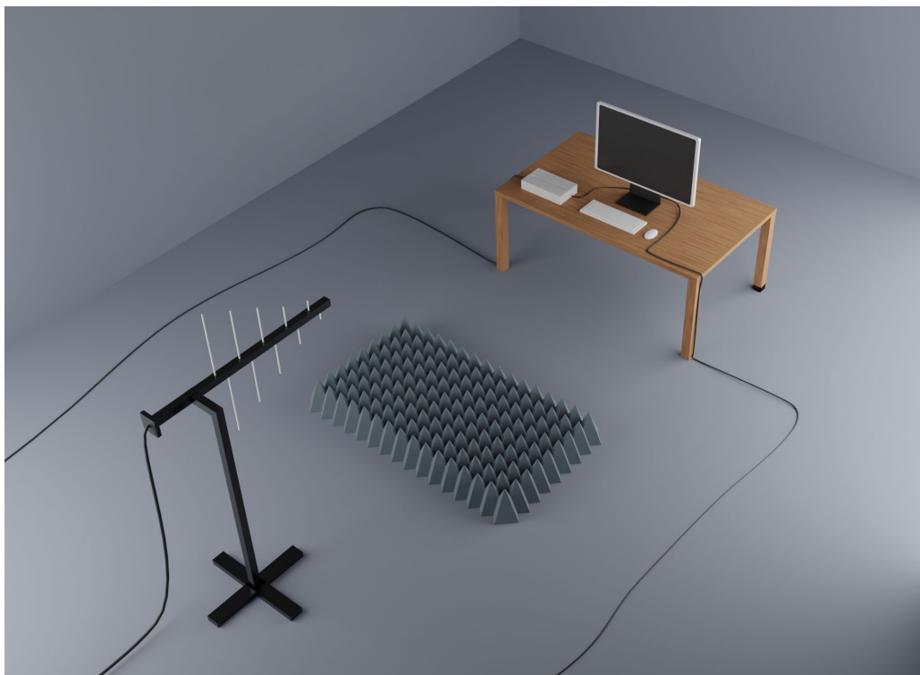
Abbildung 13: Aufbau der Störfestigkeitsprüfung gegen elektromagnetische Felder nach IEC 61000-4-3:2006+A1:2007+A2:2010
