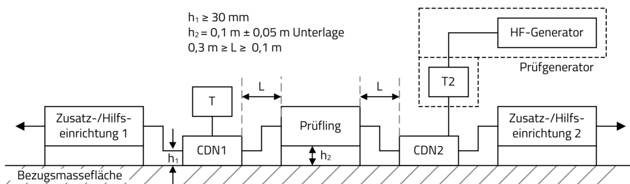
Abbildung 25: Aufbau zur Prüfung der leitungsgeföhrt Störfestigkeit nach DIN EN 61000-4-6:2014-08
