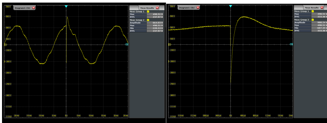
Abbildung 22: Surgeeinkopplung - 1 kV am Maximum der 230 V AC Sinusschwingung
