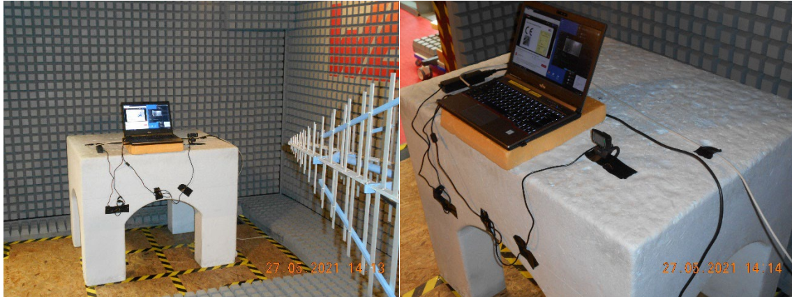
Abbildung 8: Aufbau der gestrahlten Störaussendungsprüfung des Prüflings. Verwendung eines geschirmten Ethernetkabels
